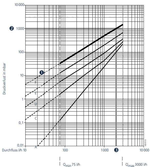
Druckverlustdiagramm Beispiel
