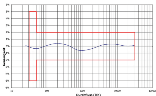
Typische Fehlerkurve – Q_3 25 m³/h
