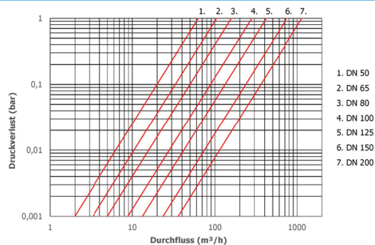
Druckverlustdiagramm
