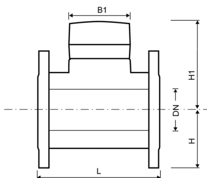
Abmessungen
