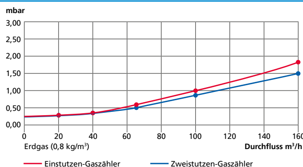
Druckverlustrdiagramm G 100
