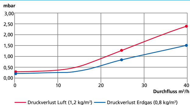
Druckverlustrdiagramm G 25
