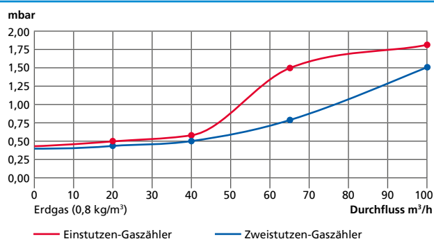
Druckverlustrdiagramm G 65
