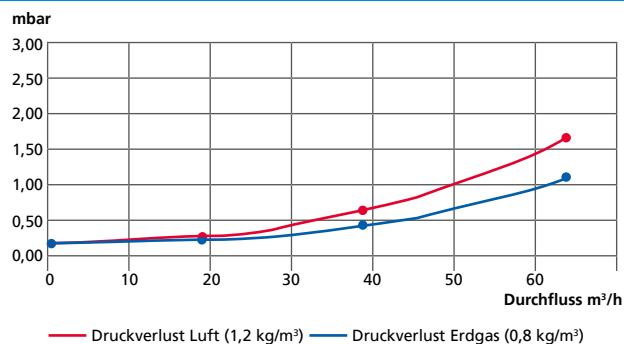
Druckverlustrdiagramm G 40
