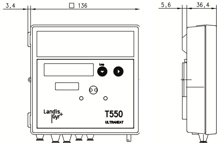
Abb. 15: Maße Rechenwerk
