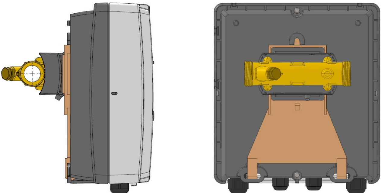
Abb. 6: MULTICAL® 803 montiert auf ULTRAFLOW® mit G\frac{3}{4} x 110 mm Gewindeanschluss mit Halterung 3026-857
