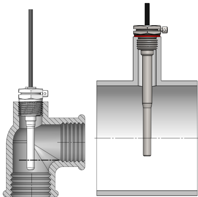
Abb. 14: Beispiele für die Montage der Tauchhülse für den Temperaturfühler ø5,8 mm mit R½-Gewinde (links) und der Tauchhülse für den Temperaturfühler ø6,0 mm mit G½-Gewinde und Kupferdichtung (rechts).
