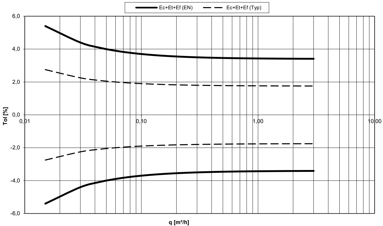
MULTICAL® 803 und ULTRAFLOW® qp 1,5 m³/h @ΔΘ 30K
