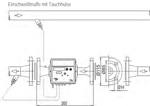
Abb. 2: Einbindung mit Tauchhülsen (empfohlen ab DN32)
