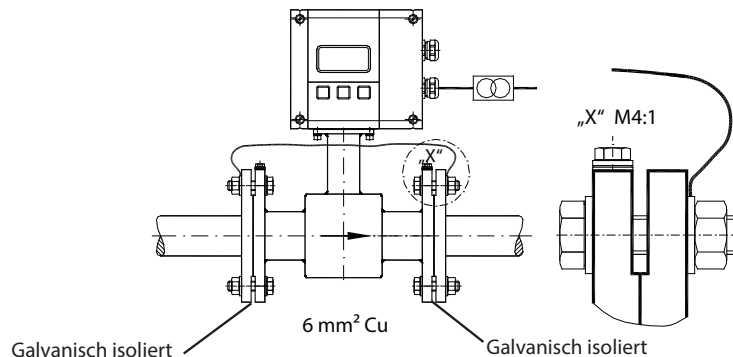
Abbildung 21: Kathodischer Schutz
