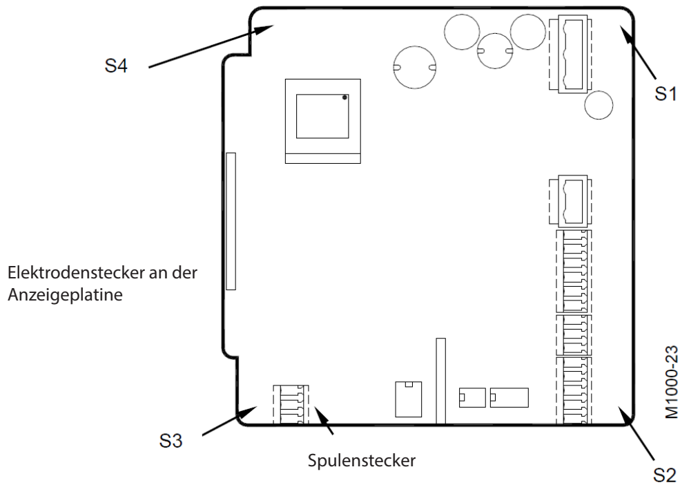
Abbildung 31: Einschraubstellen
